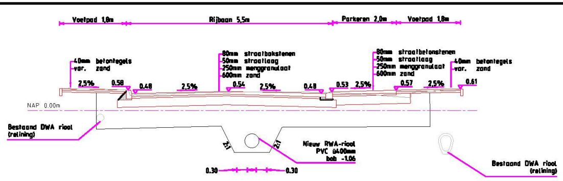
Principe dwarsdoorsnede De Buorren
